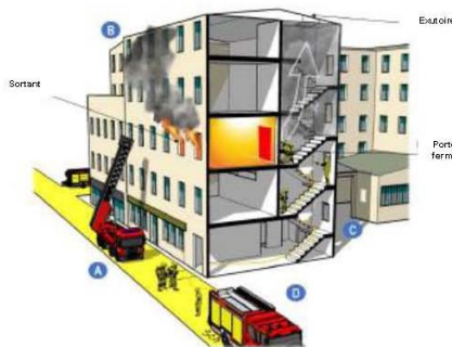
Volume non cloisonné
