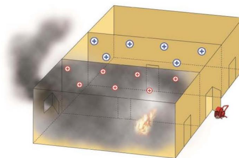
Étape n°2 : Le local contigu à protéger est mis en surpression
